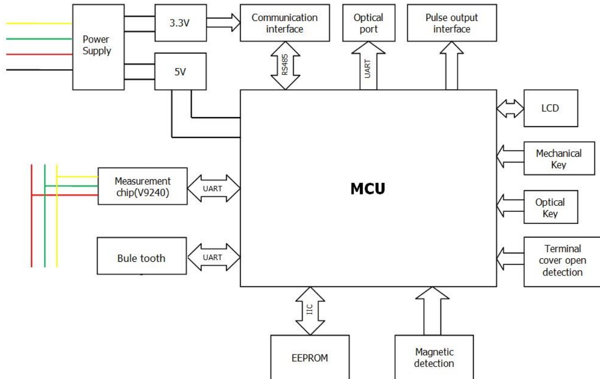
Fig. 10: Blockdiagramm
