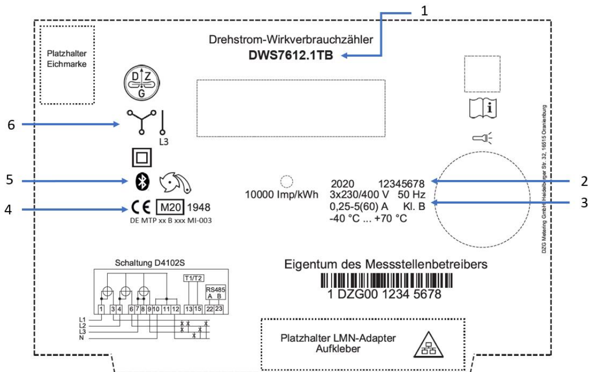
Fig. 8: Leistungsschild
