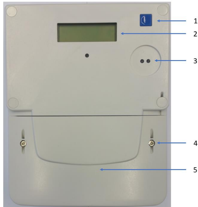
Fig. 1: Gehäuse
