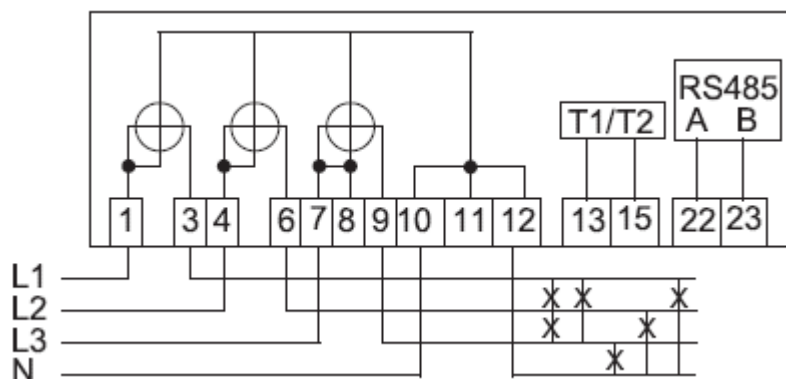
Fig. 4: Schaltbild
