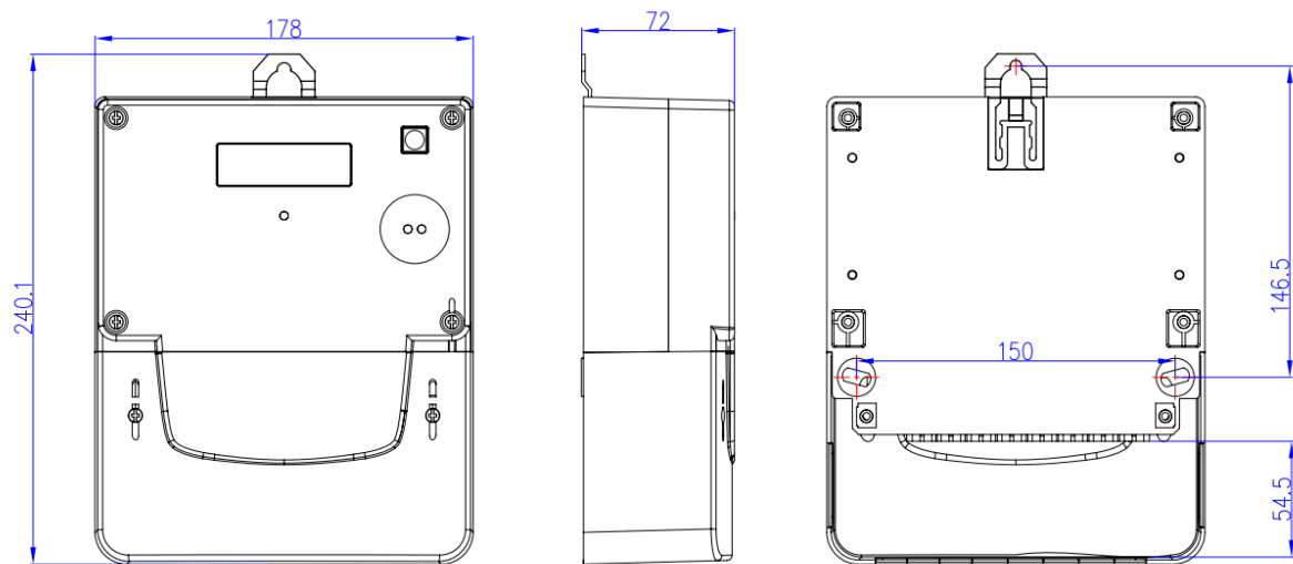
Fig. 2: Abmessungen Gehäuse
