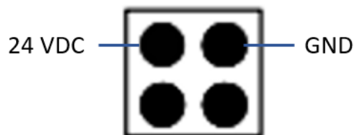
Fig. 7: Anschluss 24 VDC
