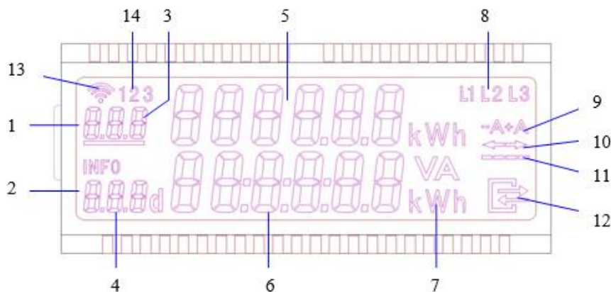
Fig. 9: LCD
